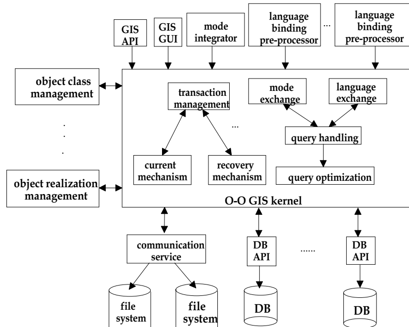
Fig. 4 GIS Structure
