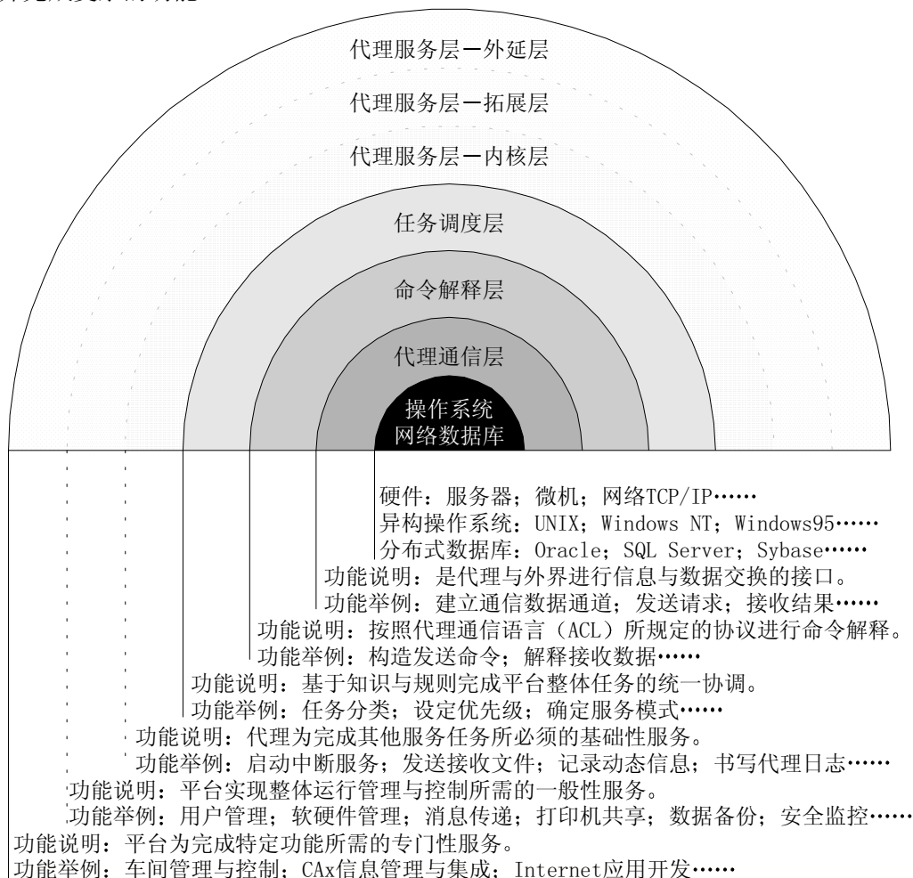
图 4. 新一代 CIMS 应用集成平台系统单元结构模型
