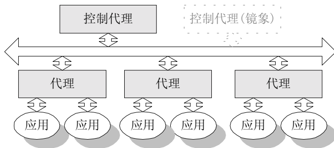
图 3. 新一代 CIMS 应用集成平台系统整体结构模型
