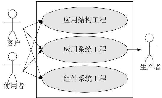
图 1. 基于重用的软件工程基本过程
