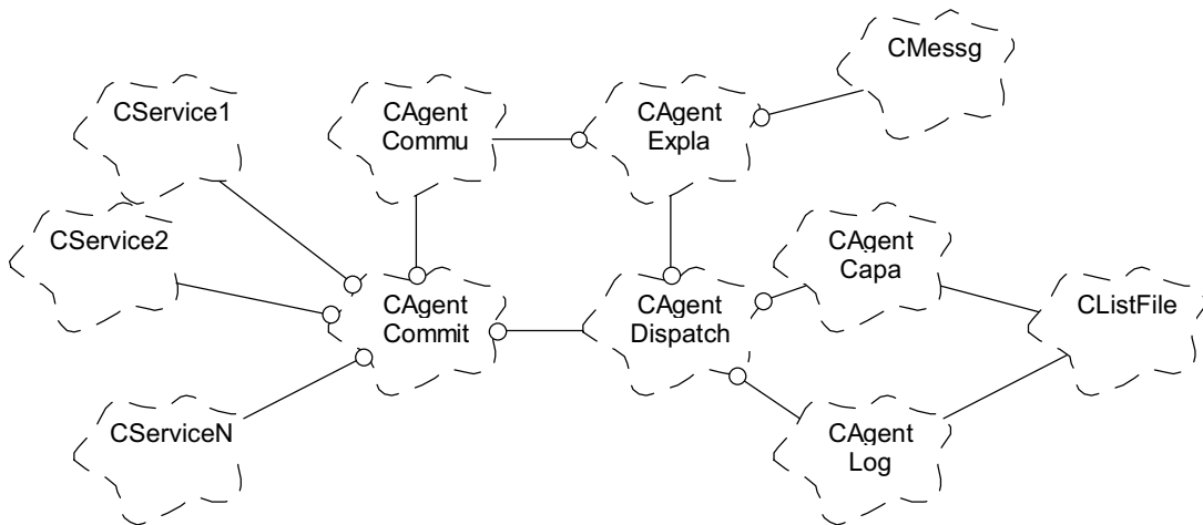
图 6. 代理的分析模型: 类图
